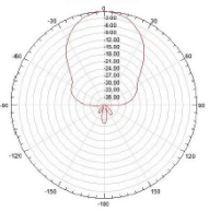
3300-3800MHz
