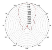
1695-2690MHz Horizontal
