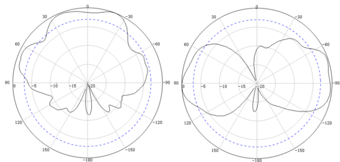
Horizontal Pattern, 2500MHz
